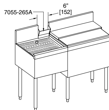
7055-265A – soda chase cutout
