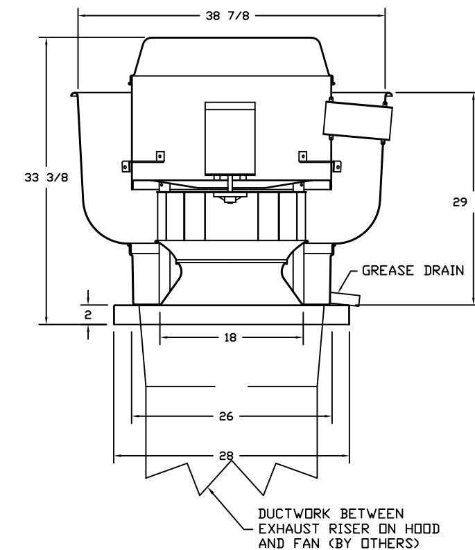
FANS #3 (EF-1), #4 (EF-1), #6 (EF-155) - DU200HFA EXHAUST FAN
