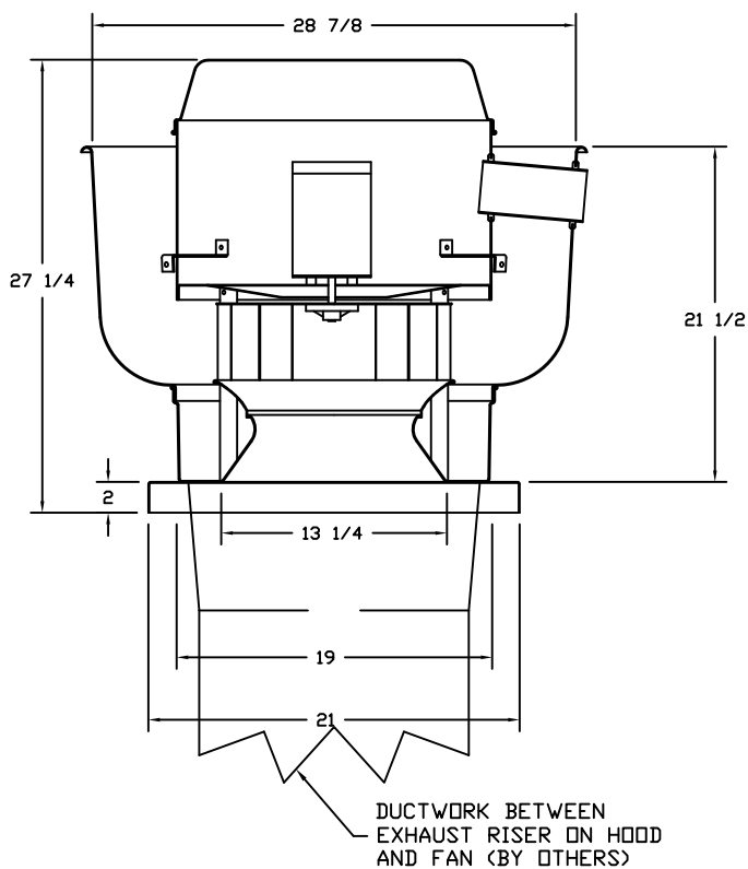
FAN #2 DU50HFA - EXHAUST FAN (EF-45)
