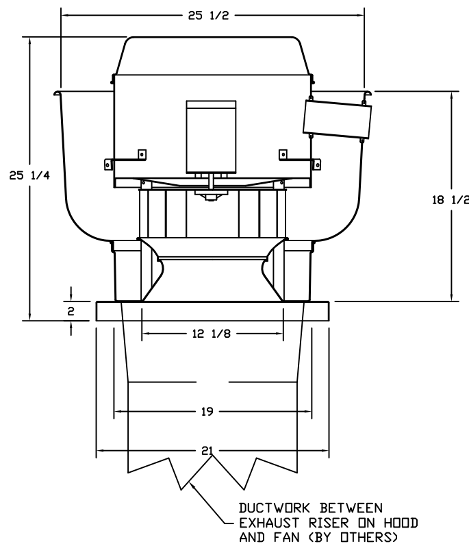
FAN #1 DU33HFA - EXHAUST FAN (EF-58)
